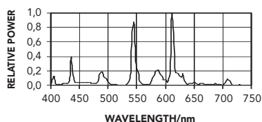
F32T8/835 HI LUMEN
